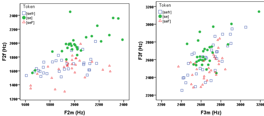
شکل ۵ و ۶: پراکندگی داده‌ها برحسب تغییرات F3 و F2 از میان به انتهای واژه /e/
